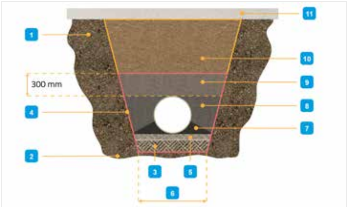
Abb. 11: Rohrgraben-Bezeichnungen
