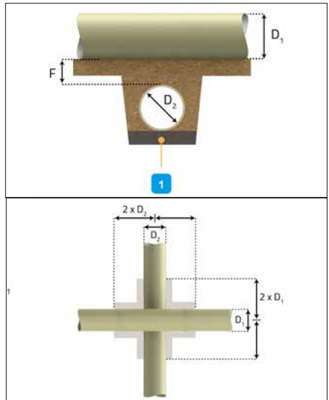
Abb. 61: Kreuzung anderer Rohrleitungen
