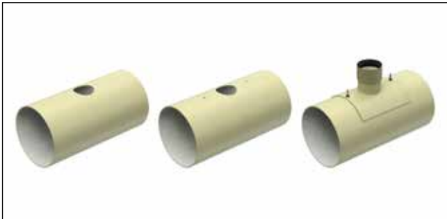
Abb. 70: Montage geschraubter Sättel
