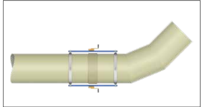
Abb. 55: Verbindung von Formstücken mit klemmbaren Montageschellen (kein Lieferumfang von Amiblu)
