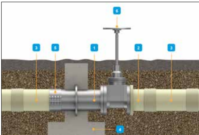
Abb. 79: Typ 2 – Widerlager neben dem Ventil
