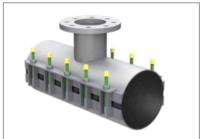
Abb. 72: Anbohrschelle
