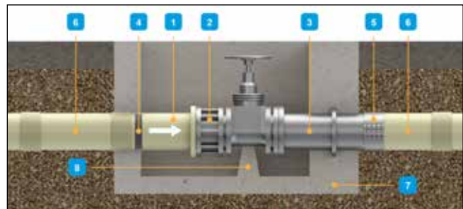
Abb. 81: Typ 4 – Verankerung mit Stahlmuerflansch
