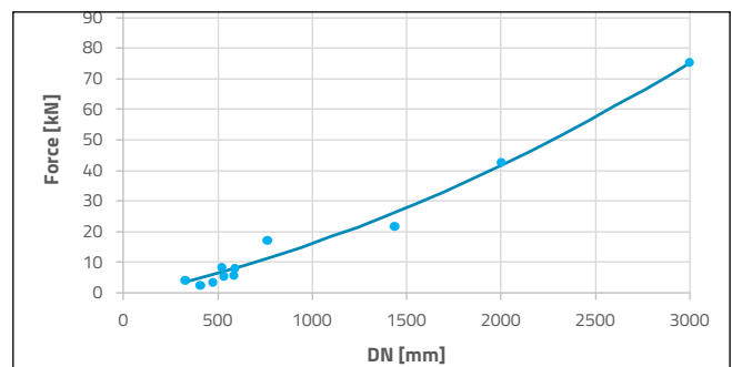
Diagramm 1: Werkseitig eingestellte Verbindungskräfte mit Kupplungen
