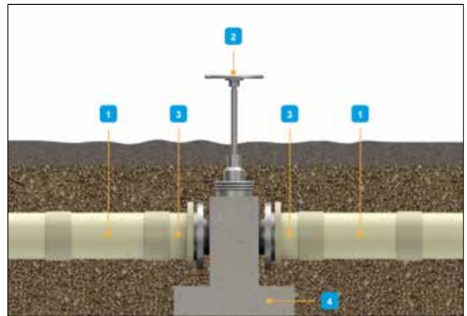
Abb. 78: Typ 1 – Armatur mit Widerlager
