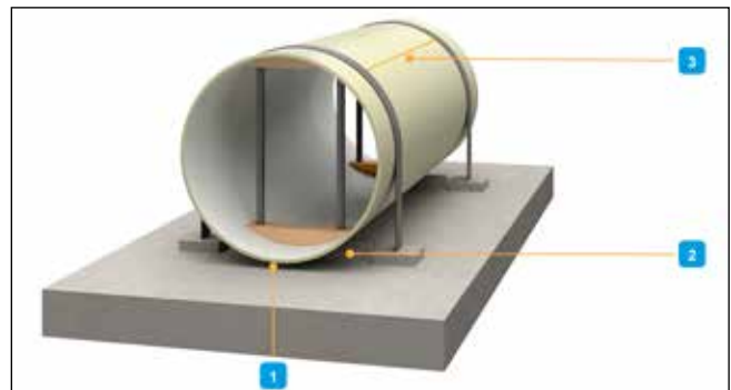
Abb. 56: Bauteilverankerung – mit innerer Aussteifung
