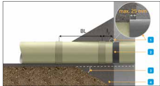
Abb. 53: Alternativer Anschluss – elastische Dichtung um einbetoniertes Rohr
