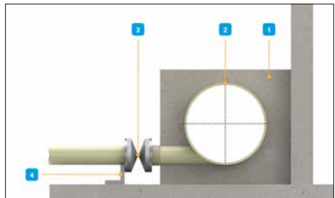
Abb. 86: Anordnung einer Entleerung
