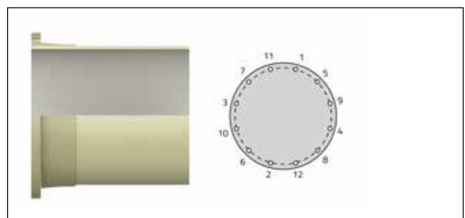
Abb. 37: Festflansch
