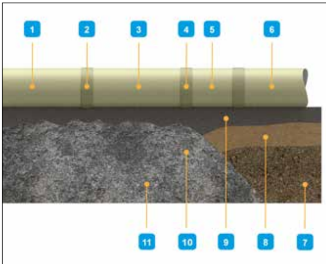
Abb. 63: Methode zum Grabenbau und zur Rohrverlegung an einem Fels-Boden-Übergang 1
