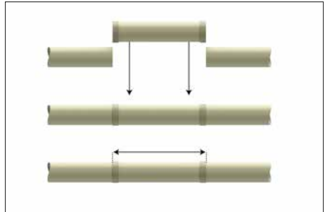
Abb. 67: Montage des Passrohres
