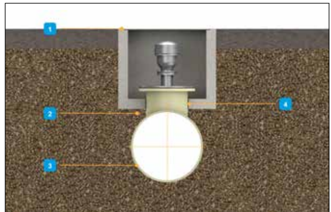
Abb. 84: Übliche Anordnung eines großen Be- und Entlüftungsventiles auf einem Amiblu T-Stück
