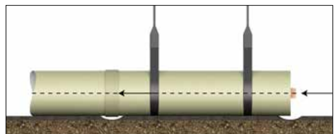
Abb. 35: Rohrverbindung mit geeigneter Ausrüstung (Schlingen nicht unbedingt erforderlich)
