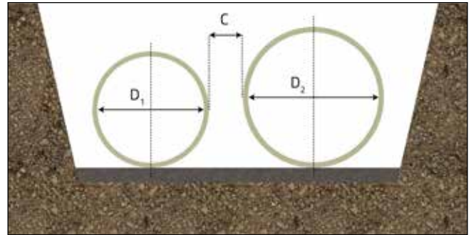
Abb. 60: Mindestabstand (C) zwischen Rohrleitungen
