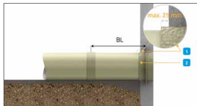
Abb. 52: Anschluss an Gebäude mit Mauerwerkskupplung
