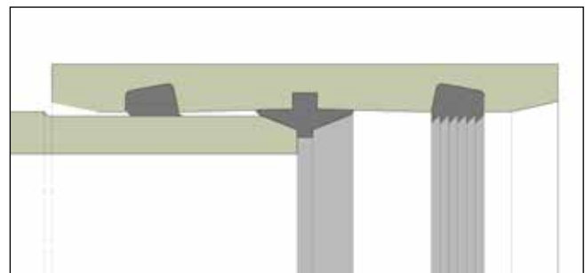
Abb. 24: FPCA-Kupplung für Druckerwendungen
