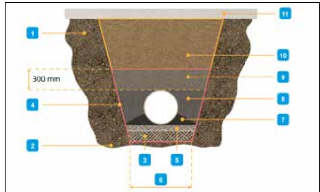
Abb. 11: Rohrgraben-Terminologie
