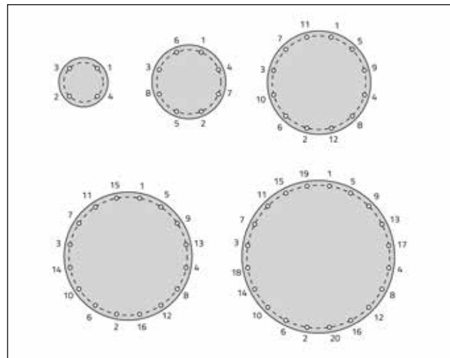
Abb. 46: Anzugsreihenfolgen
