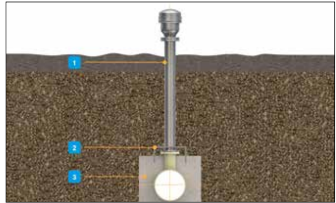
Abb. 83: Stützblock für große Verlegetiefen
