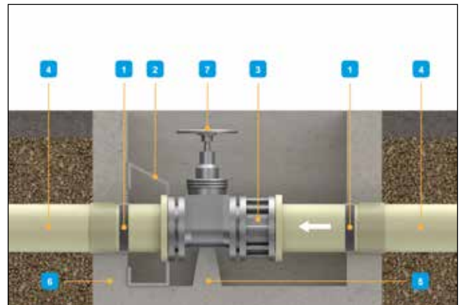
Abb. 80: Typ 3 – Widerlager neben dem Ventil
