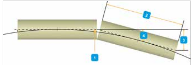
Abb. 34: Systemdarstellung Kupplungsabwinklung
