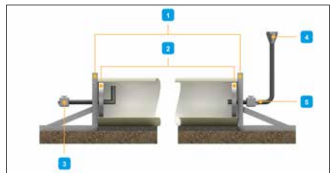
Abb. 64: Temporäres Ventil für den Dichtigkeitstest von Rohrleitungsabschnitten
