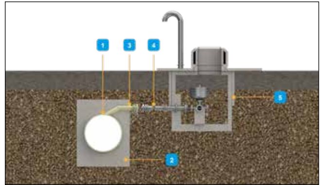
Abb. 85: Alternative Methode zur Anordnung eines großen Be- und Entlüftungsventiles im seitlichen Schacht
